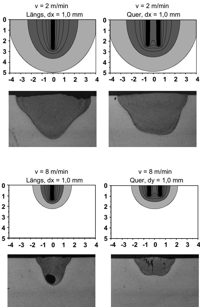
Bild 76: Vergleich der Schweißnahtgeometrie aus Rechnung und Experiment [94] bei verschiedenen Schweißgeschwindigkeiten (2 m/min, 8 m/min) mit Längs- und Queranordnung bei dem Fokiabstand ds = 1,0 mm für AlMgSi 1.
