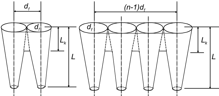
Bild 25: Teilweise getrennte Kapillargeometrie bei der Mehrfokustechnik.
