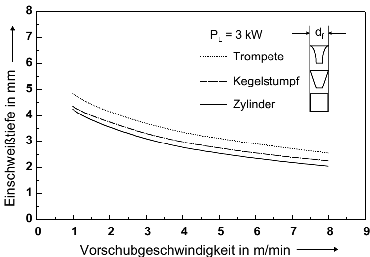
Bild 56: Einfluß der Kapillargeometrie auf die Einschweißtiefe bei Einstrahlschweißtechnik in Abhängigkeit von der Vorschubgeschwindigkeit bei gleichem Fokusbereich d_f = 0,3 \text{ mm} auf der Werkstückoberfläche, AlMgSi 1.
