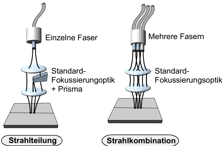
Bild 3: Methoden zur Realisierung von Mehrfokustechnik [54].
