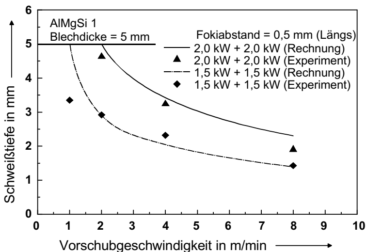
Bild 72: Vergleich der Schweißergebnisse von Rechnung und Experiment für unterschiedliche Leistung, dx = 0,5 mm, d_f = 0,3 mm, AlMgSi 1.
