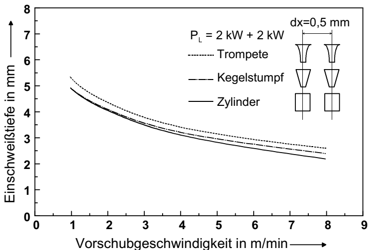
Bild 57: Einfluß der Kapillargeometrie auf die Einschweißtiefe bei Mehrfokusschweißtechnik in Abhängigkeit von Vorschubgeschwindigkeit bei gleichem Fokusbereich d_f = 0,3 \text{ mm} auf der Werkstückoberfläche, dx = 0,5 \text{ mm} , AlMgSi 1.
