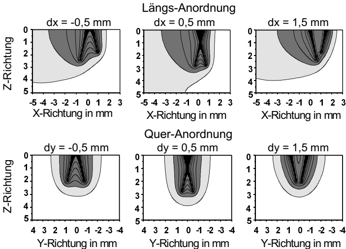
Bild 54: Temperaturverteilungen und Schmelzbadkonturen bei variiertem Fokiabstand und verschiedener Strahlanordnung. Das negative Vorzeichen des Fokiabstands bedeutet zwei nach außen gerichtete Laserstrahlen; P_L = 2 \text{ kW} + 2 \text{ kW} , d_f = 0,3 \text{ mm} , v = 4 \text{ m/min} .
