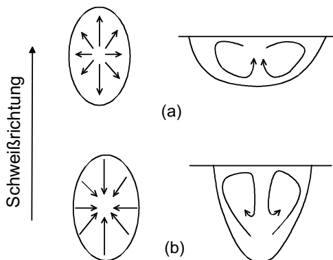
Bild 7: Marangoni-Strömung im Schmelzbad, (a): Negativer Oberflächenspannungsgradient \frac{d\sigma}{dT} < 0 , (b): Positiver Oberflächenspannungsgradient \frac{d\sigma}{dT} > 0 [70].
