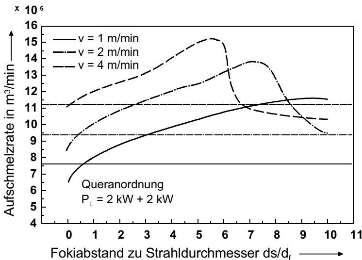
Bild 108: Aufschmelzrate (Produkt von Nahtfläche und Geschwindigkeit) über dem normierten Fokidabstand bei verschiedenen Schweißgeschwindigkeiten für Stahl; Zweistrahltechnik in Queranordnung.
