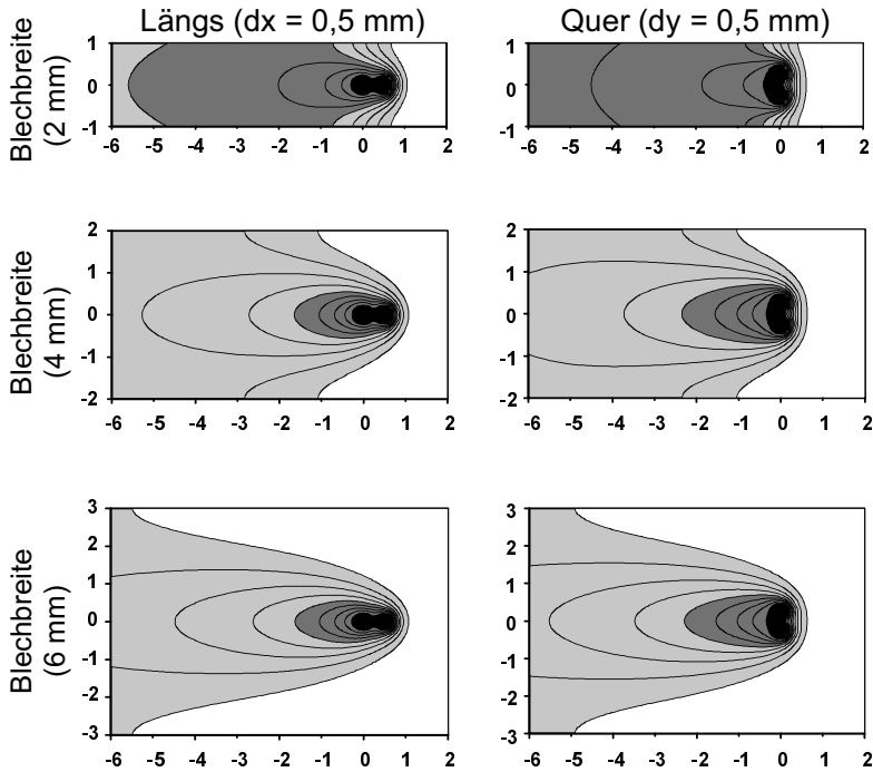
Bild 84: Grenzeffekt für unterschiedliche Blechbreiten bei Variation der Fokianordnungen, v = 4 \text{ m/min} , Stahl, Einschweißung im halbunendlichen Körper.
