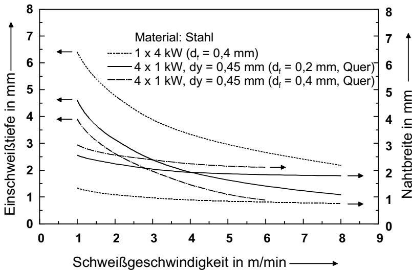
Bild 42: Berechnete Schweißergebnisse für die Ein- und Mehrfokustechnik mit verschiedenen Fokusdurchmessern (Stahl, v = 4 \text{ m/min} ).
