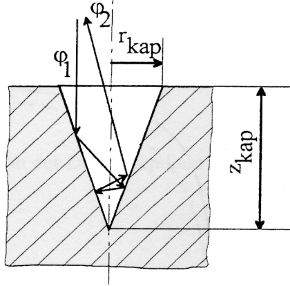
Bild 16: Berechnung des Einkoppelgrades mit kegelförmig angenäherte Kapillare [32].
